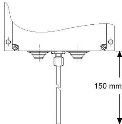
Fig. 6 Style 28 Raccord à souder 6 mm ODM
