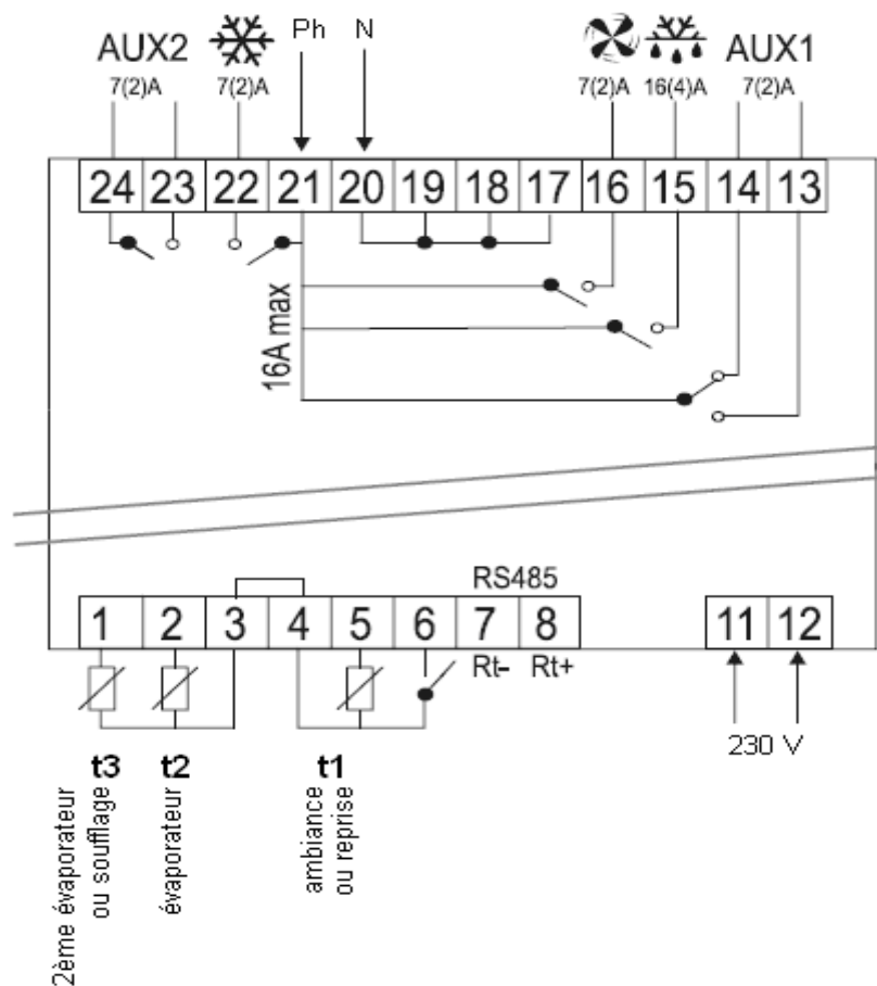
Figure 6 : Schéma de câblage
