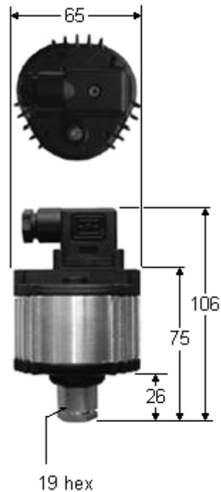
Style 47 7/16 -20 UNF femelle (avec poussoir Schrader)
