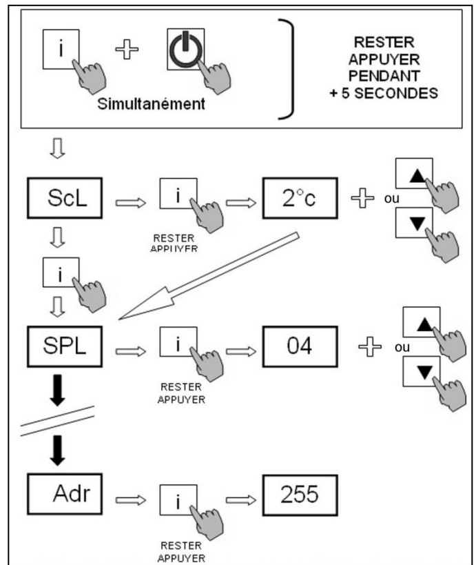
Fig. 5 Réglage des Paramètres (Voir liste)
