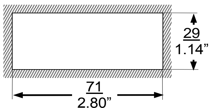
Fig. 6 Découpe du panneau
