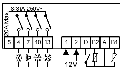
Schéma de câblage a)
