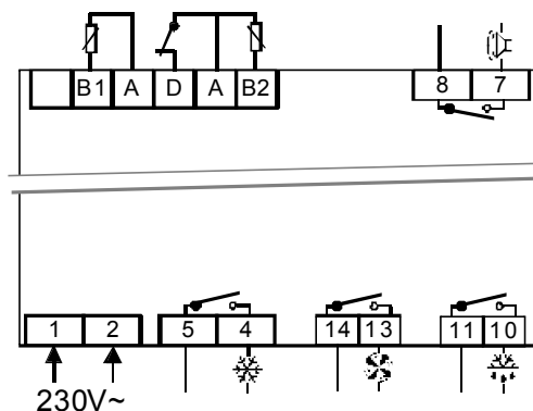
Schéma de câblage b)
