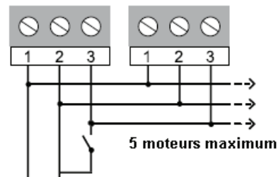
Figure 6 : M9108-ADx et AGx (Signal Tout ou Rien)
