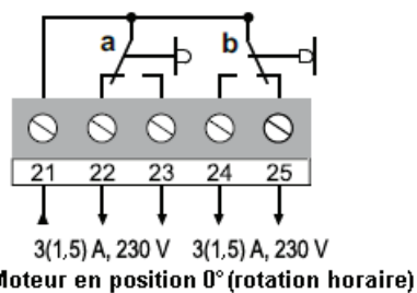
Figure 8 : M9108ADC, AGC et GGC
